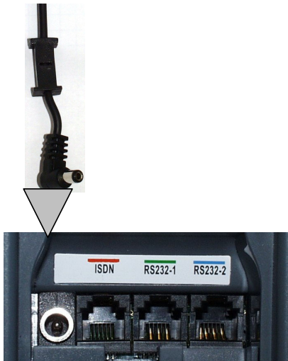
Abbildung 4 - Stromversorgung
