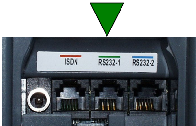
Abbildung 5 - Anschluss Kasse
